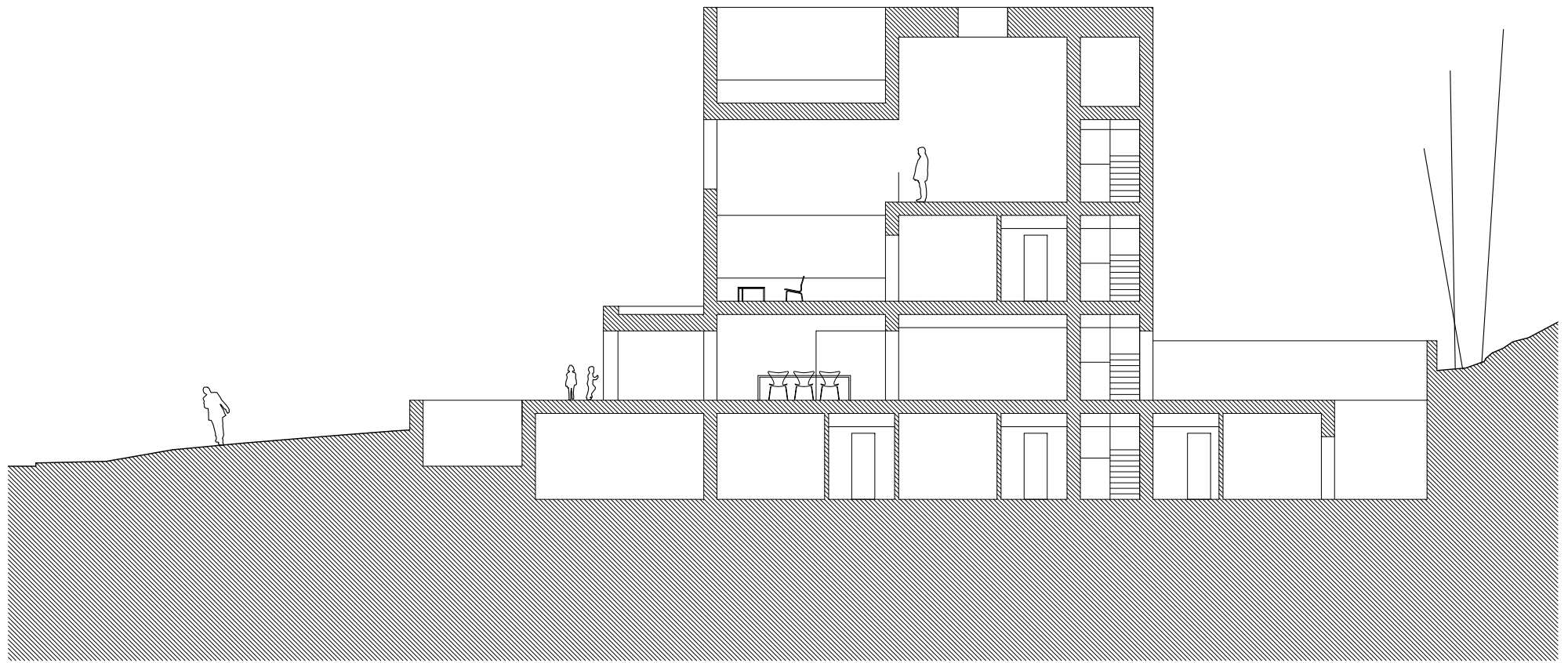
LONGITUDINAL SECTION
