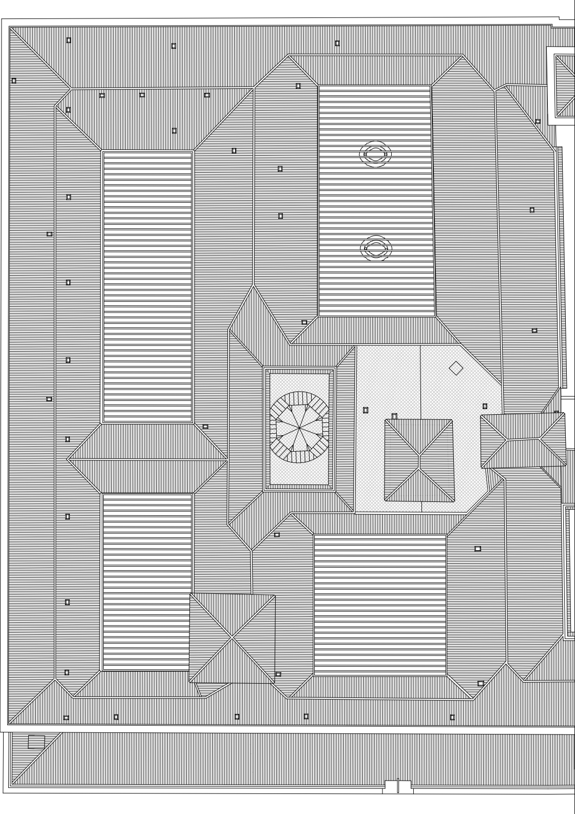
PLANTA CUBIERTA PROYECTO
