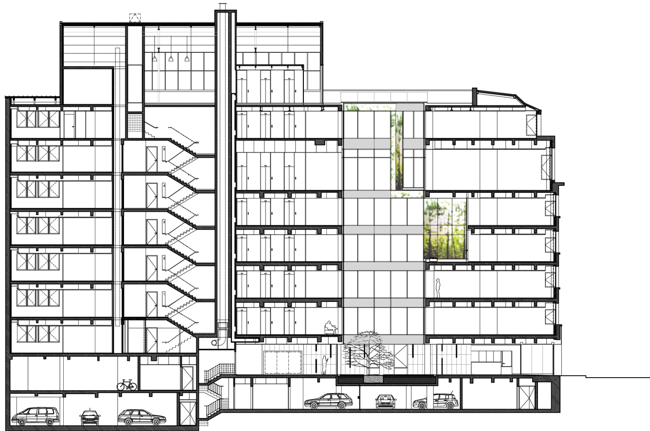
COUPE LONGITUDINALE // ATELIERS 2/3/4/
