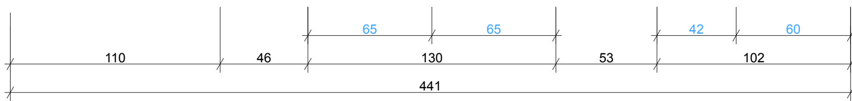
SCHNITT A-A
