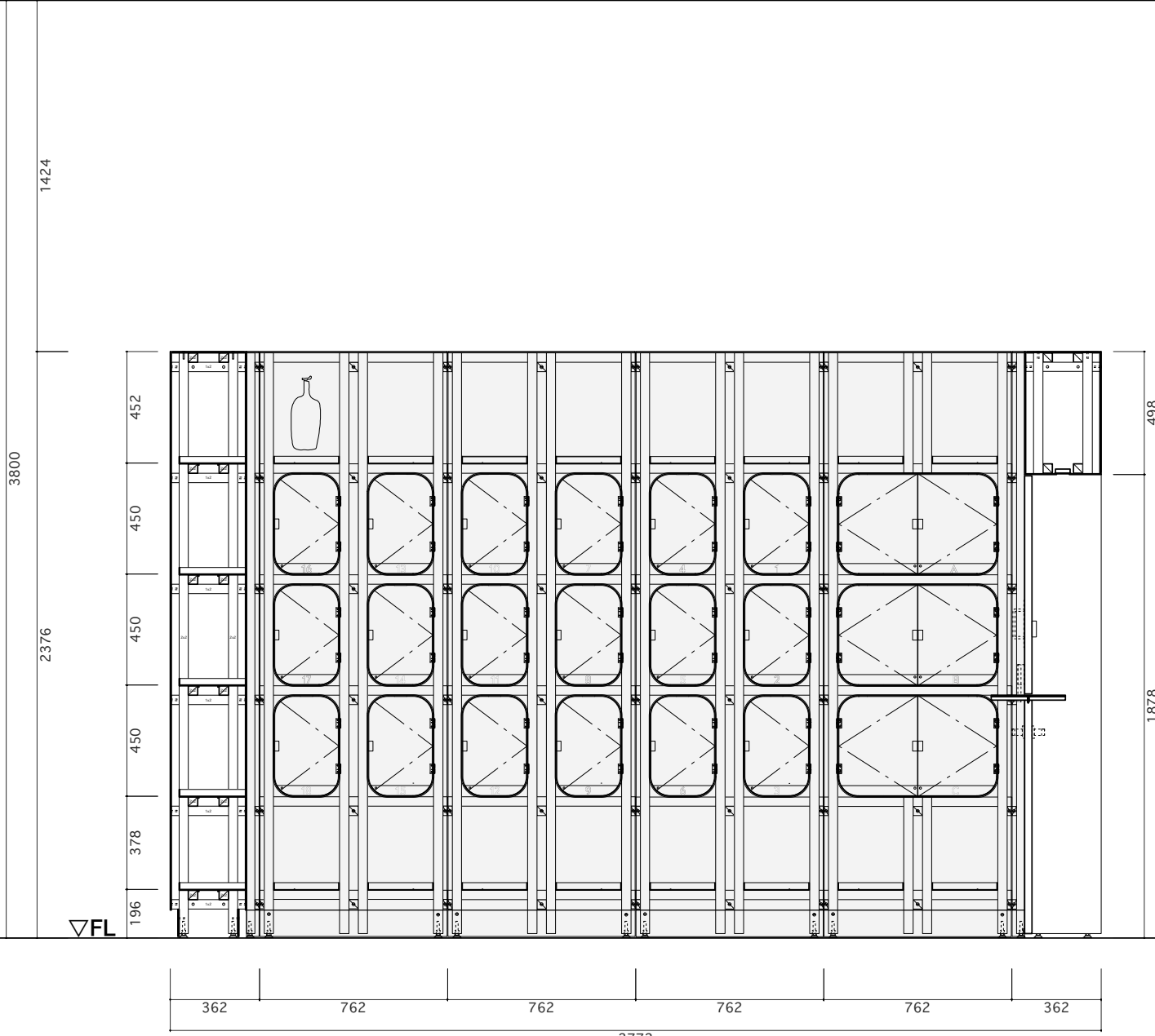
Section A-A'
