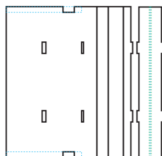
1ud Estante inferior Aviplex 9,3mm
