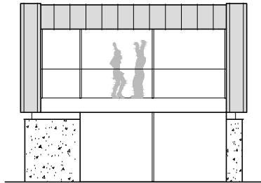
PROSPETTO OVEST
