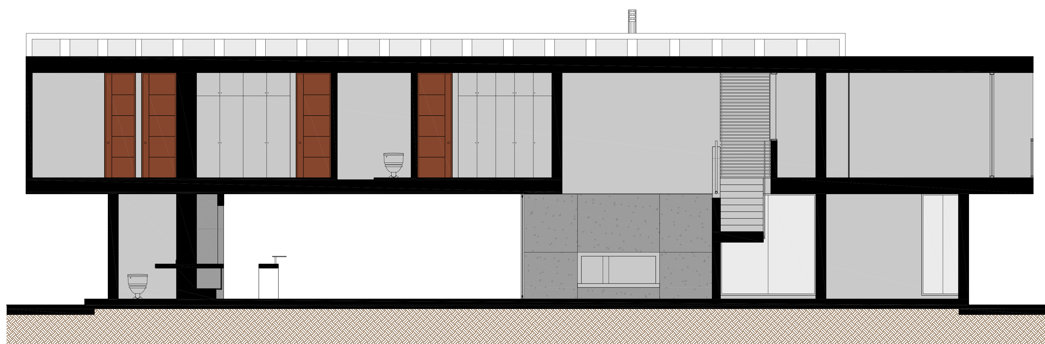
CORTE A-A
