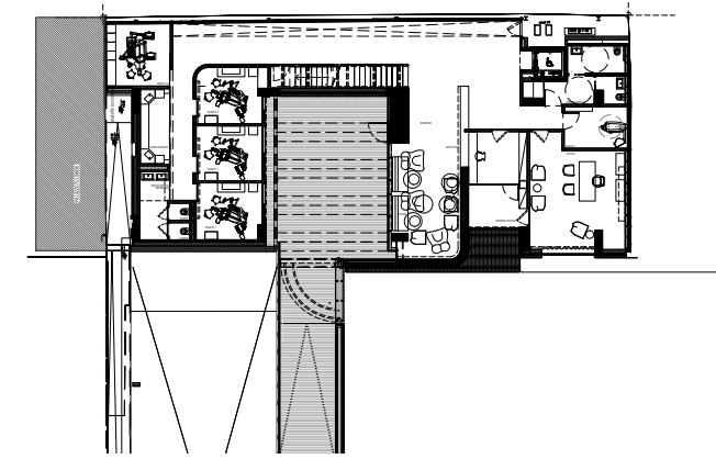
Piano primo
