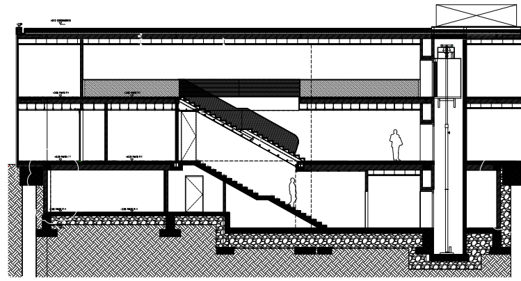
Sezione longitudinale
