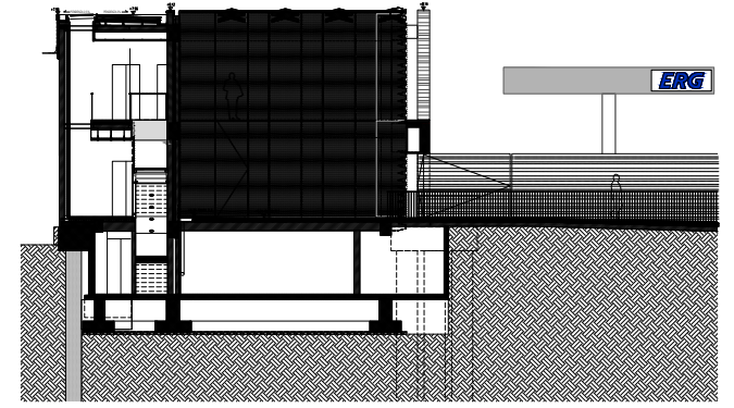
Sezione trasversale
