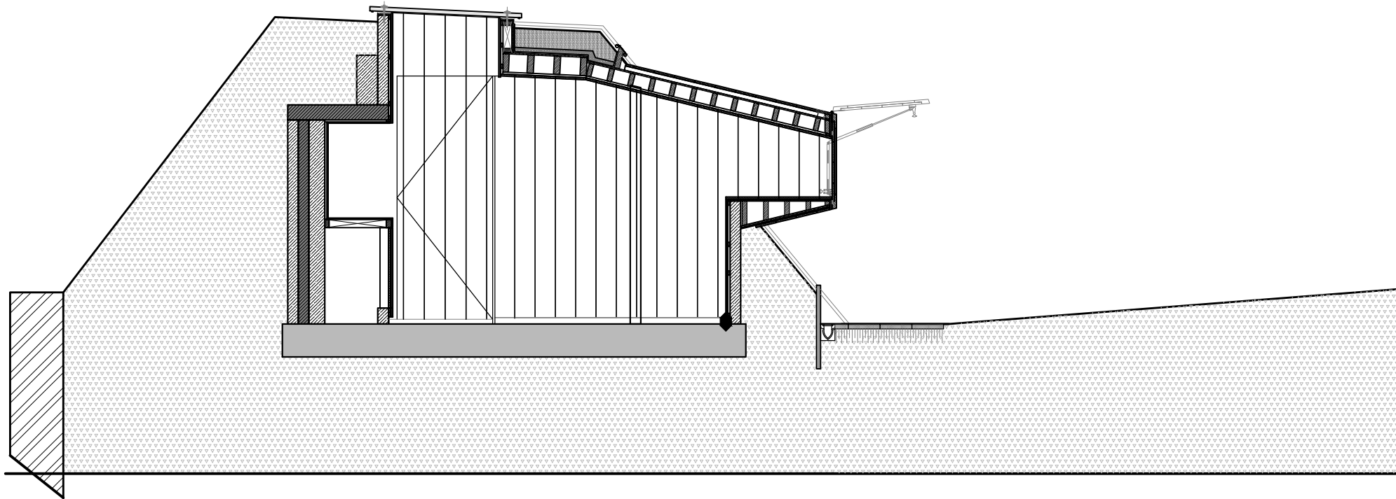
doorsnede BB
