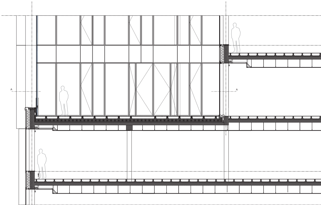
COUPE 1-1
