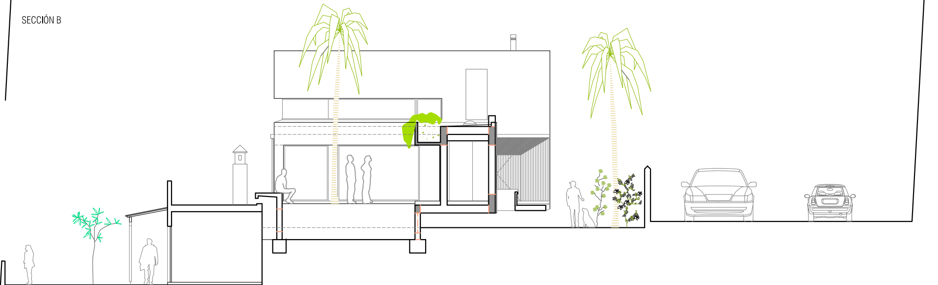
SECCIÓN A
