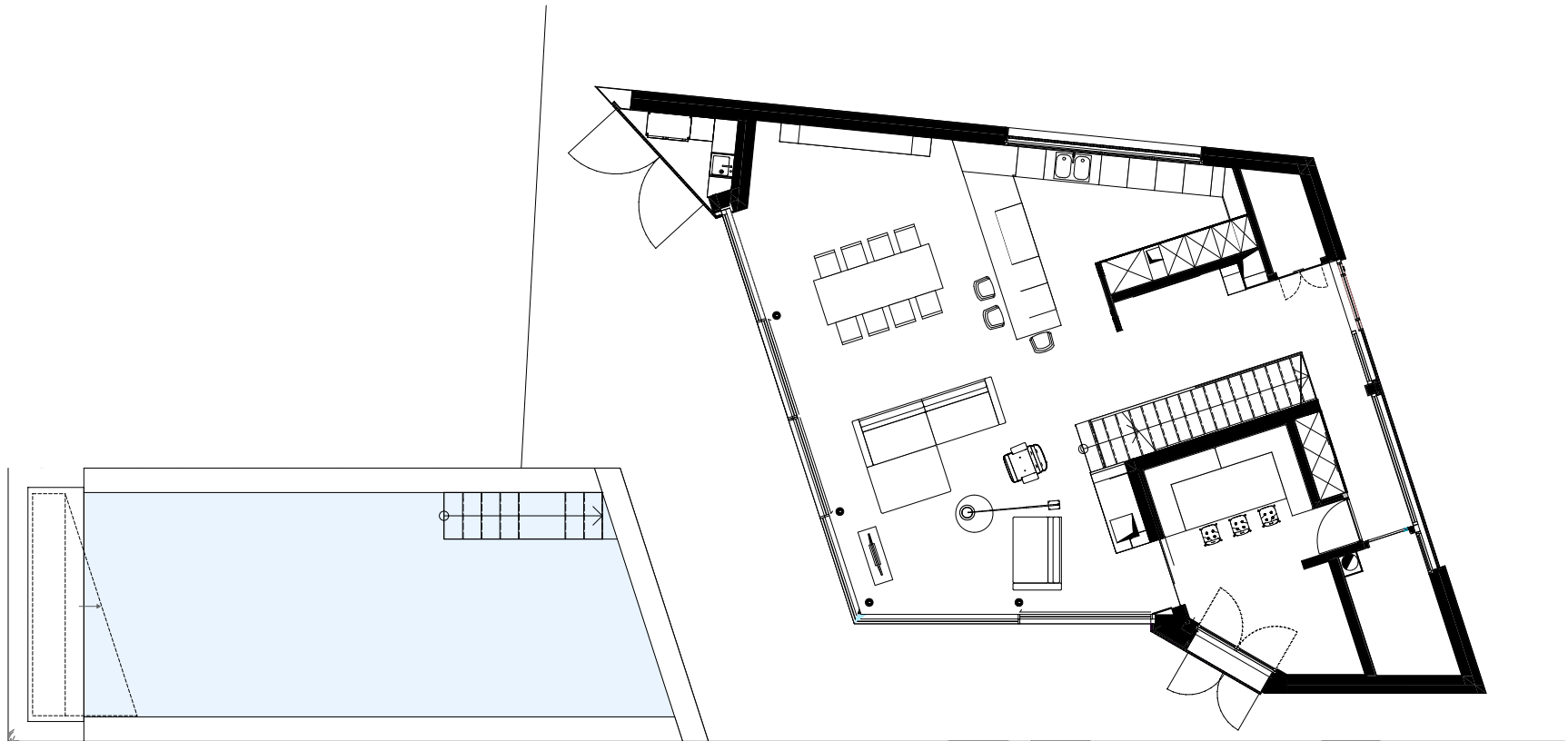
Grundriss Erdgeschoss M 1:100
