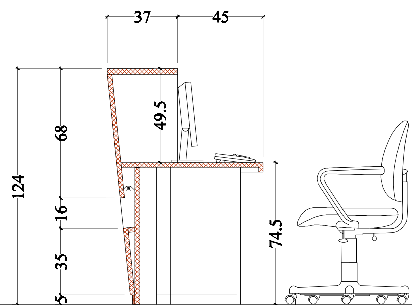
SEZIONE A-A'
