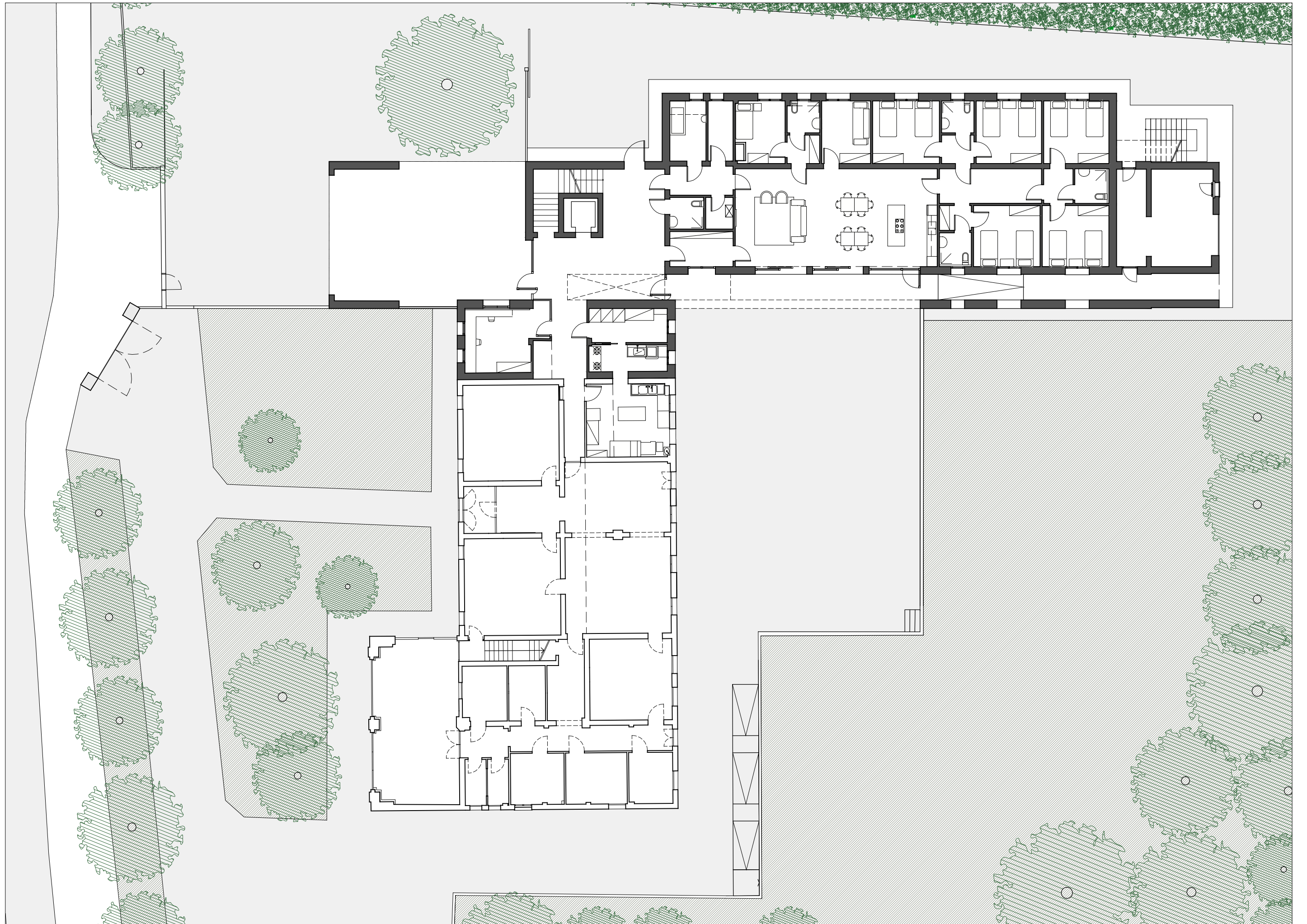
PLANIMETRIA PIANO TERRA | scala 1:200
