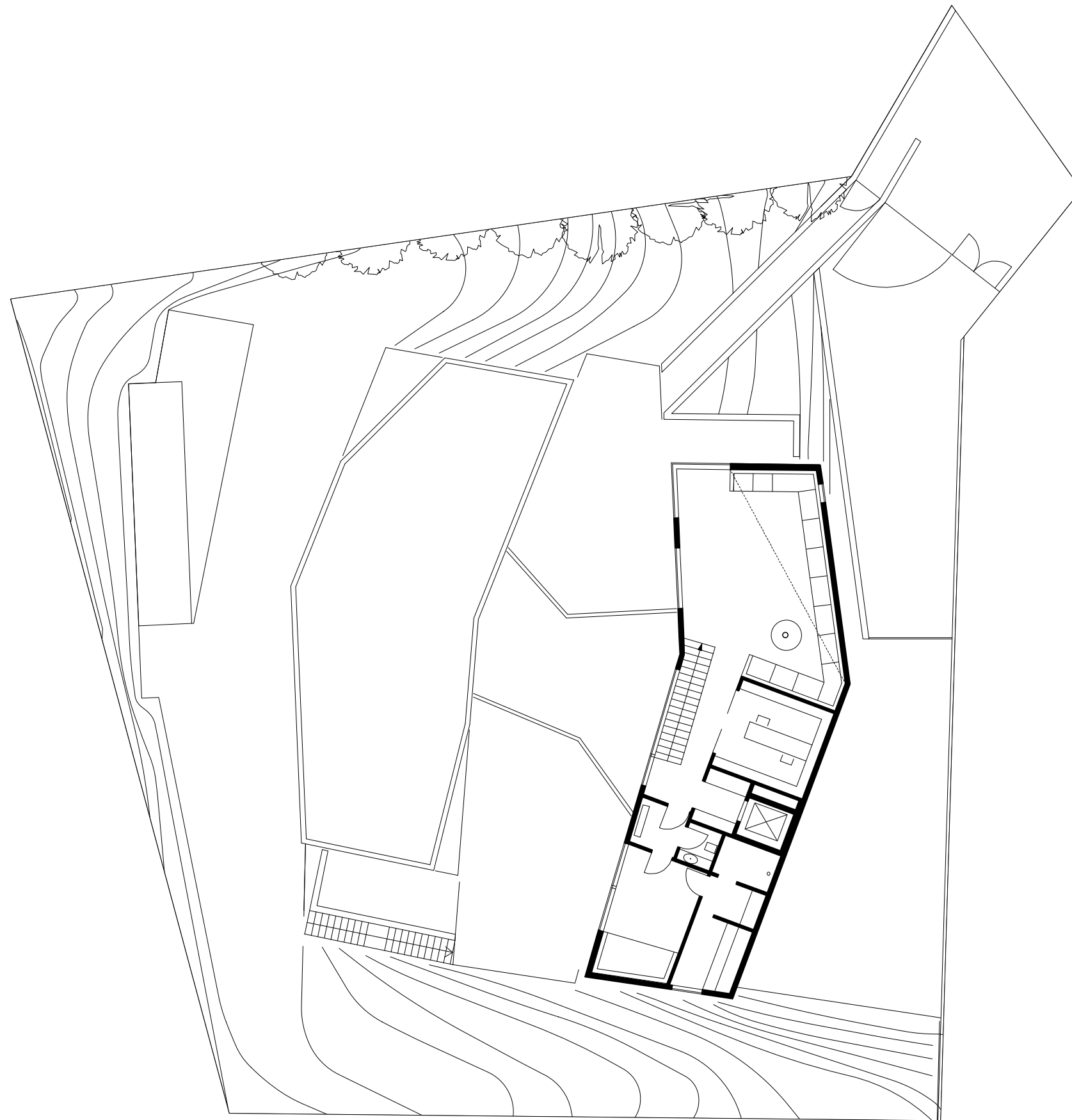
Obergeschoss M 1:200
