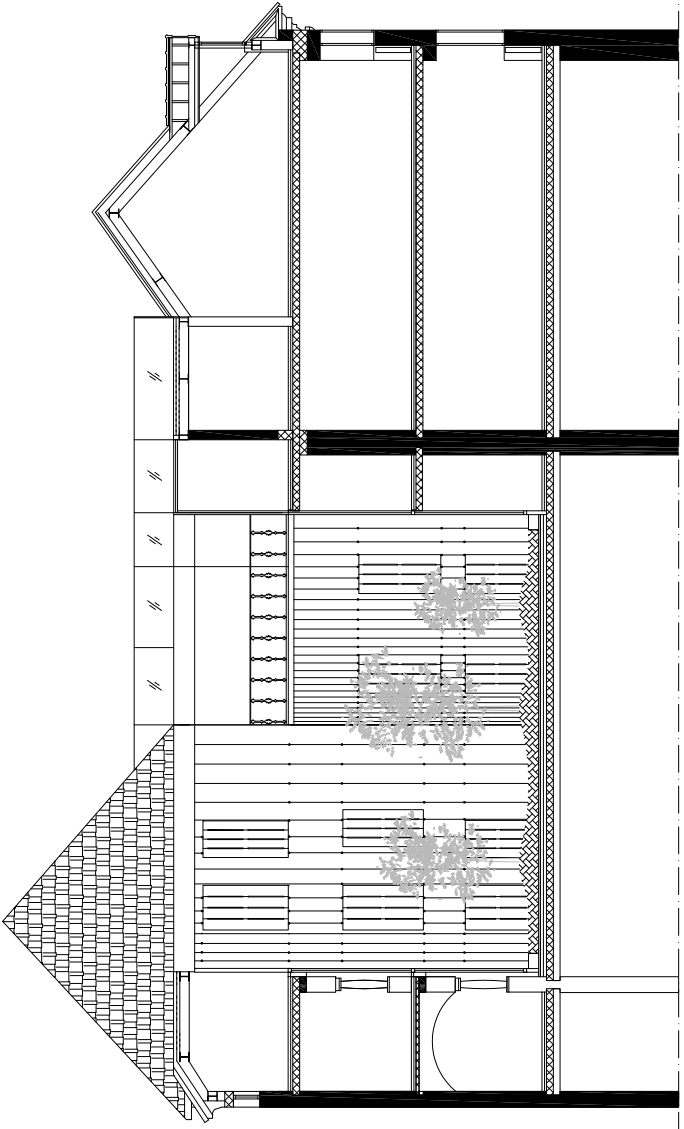
SECTION A-A
