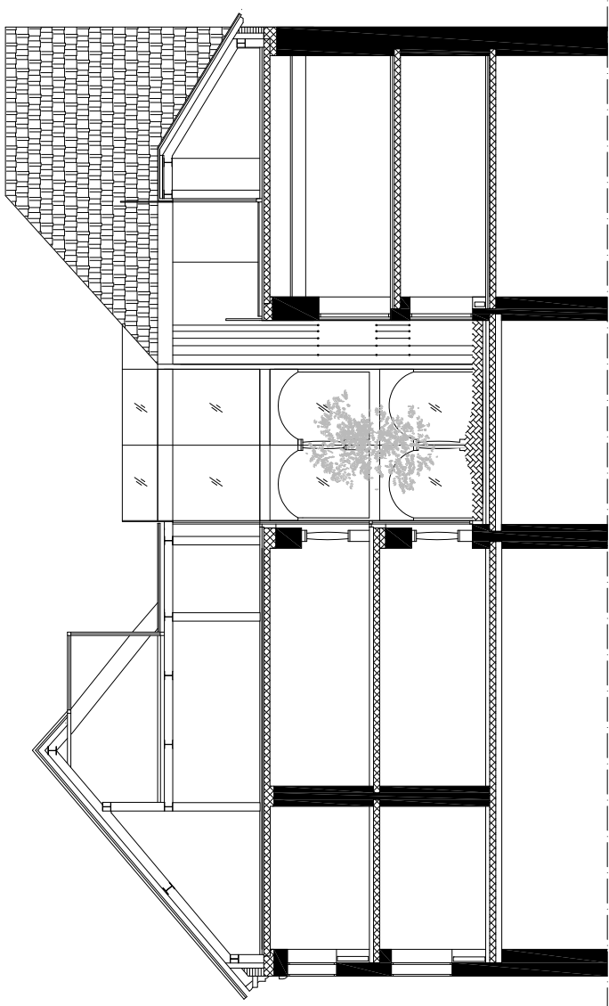
SECTION D-D
