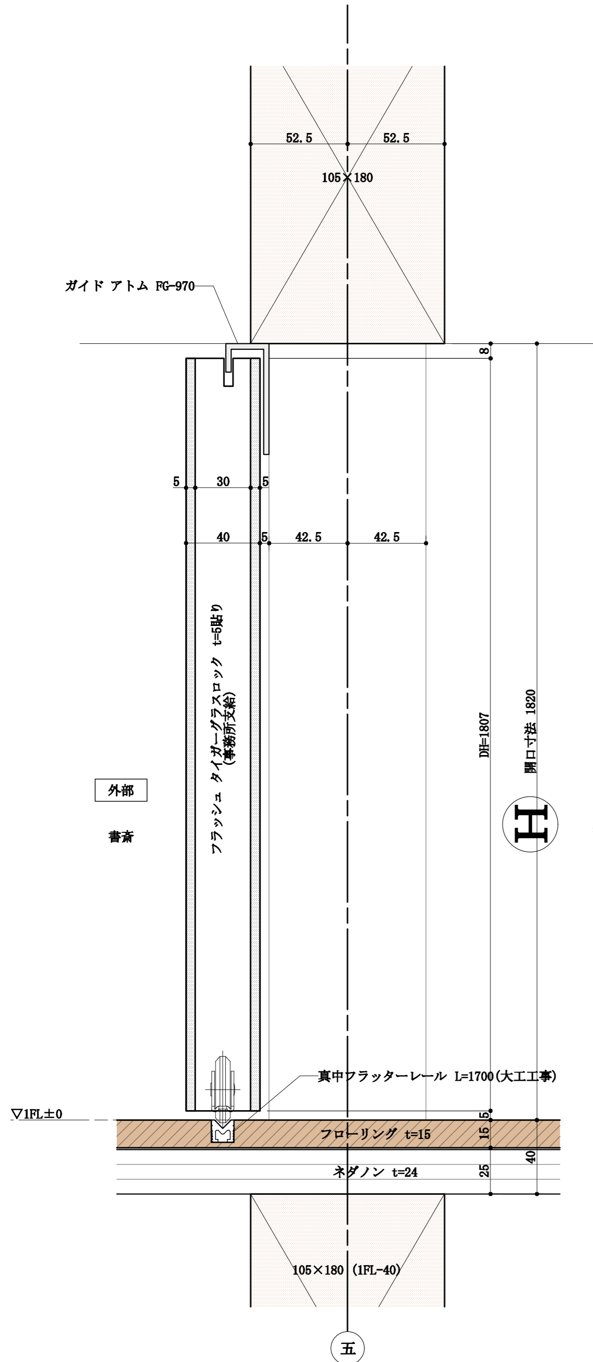
FD-2 断面詳細図 1:2
