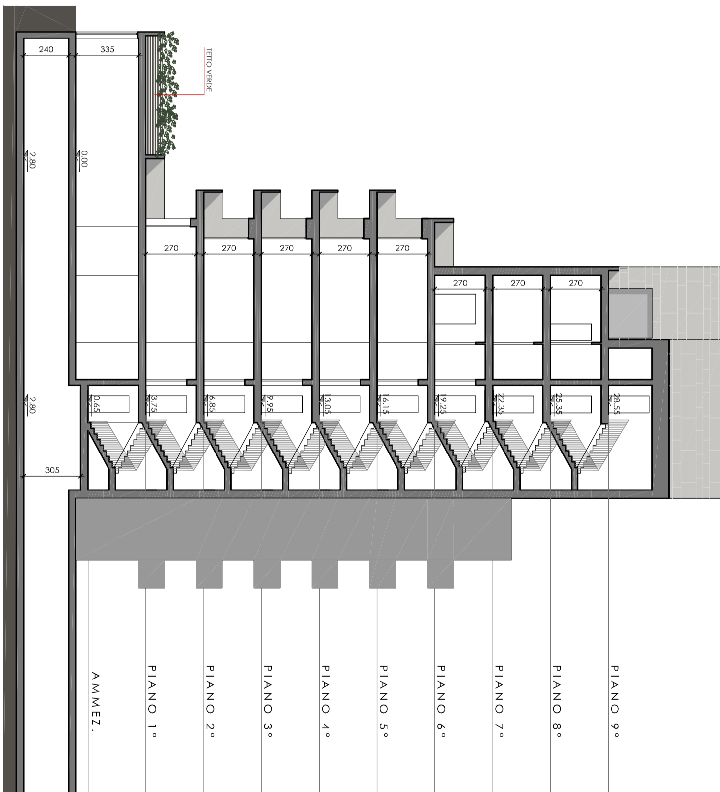
PROGETTO DI EDIFICIO RESIDENZIALE CON SPAZI COMMERCIALI AL PIANO TERRA Via Friuli - Venezia Giulia 5 - Bologna
