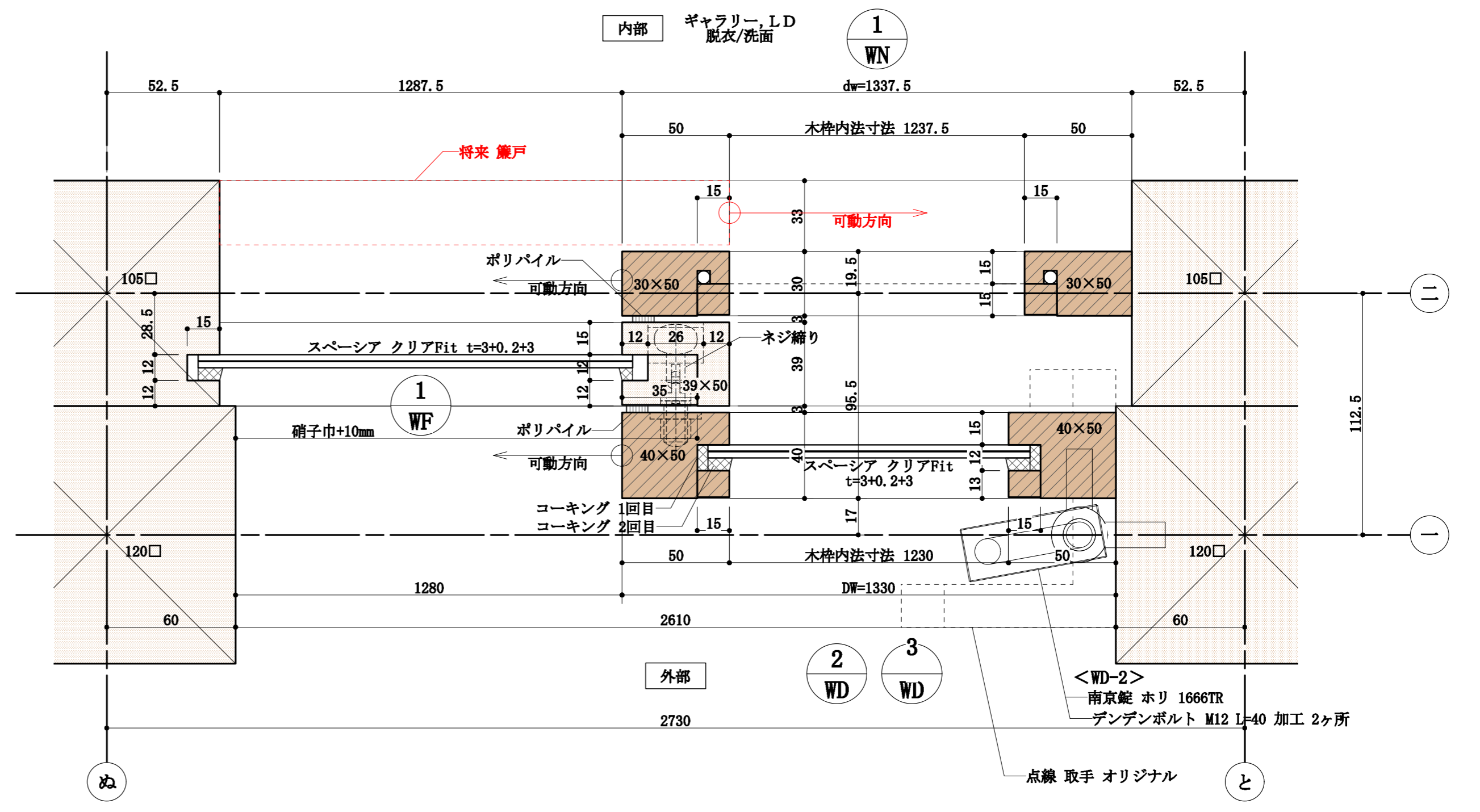
WD-2,3,WF-1,WN-1 平面詳細図 1:2
