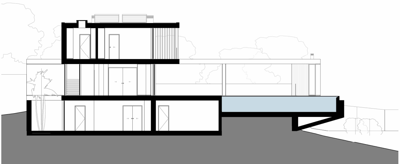
CORTE 6
