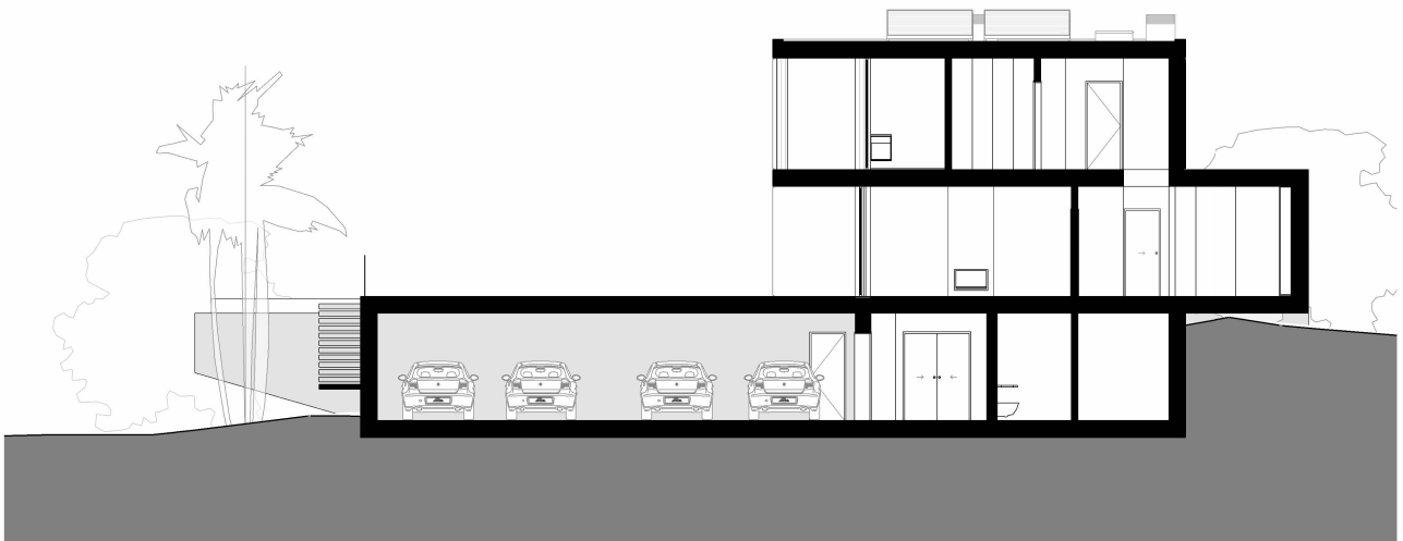
CORTE 5
