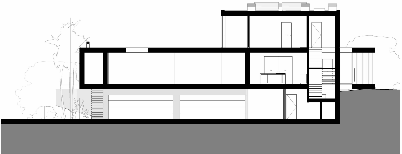
CORTE 4
