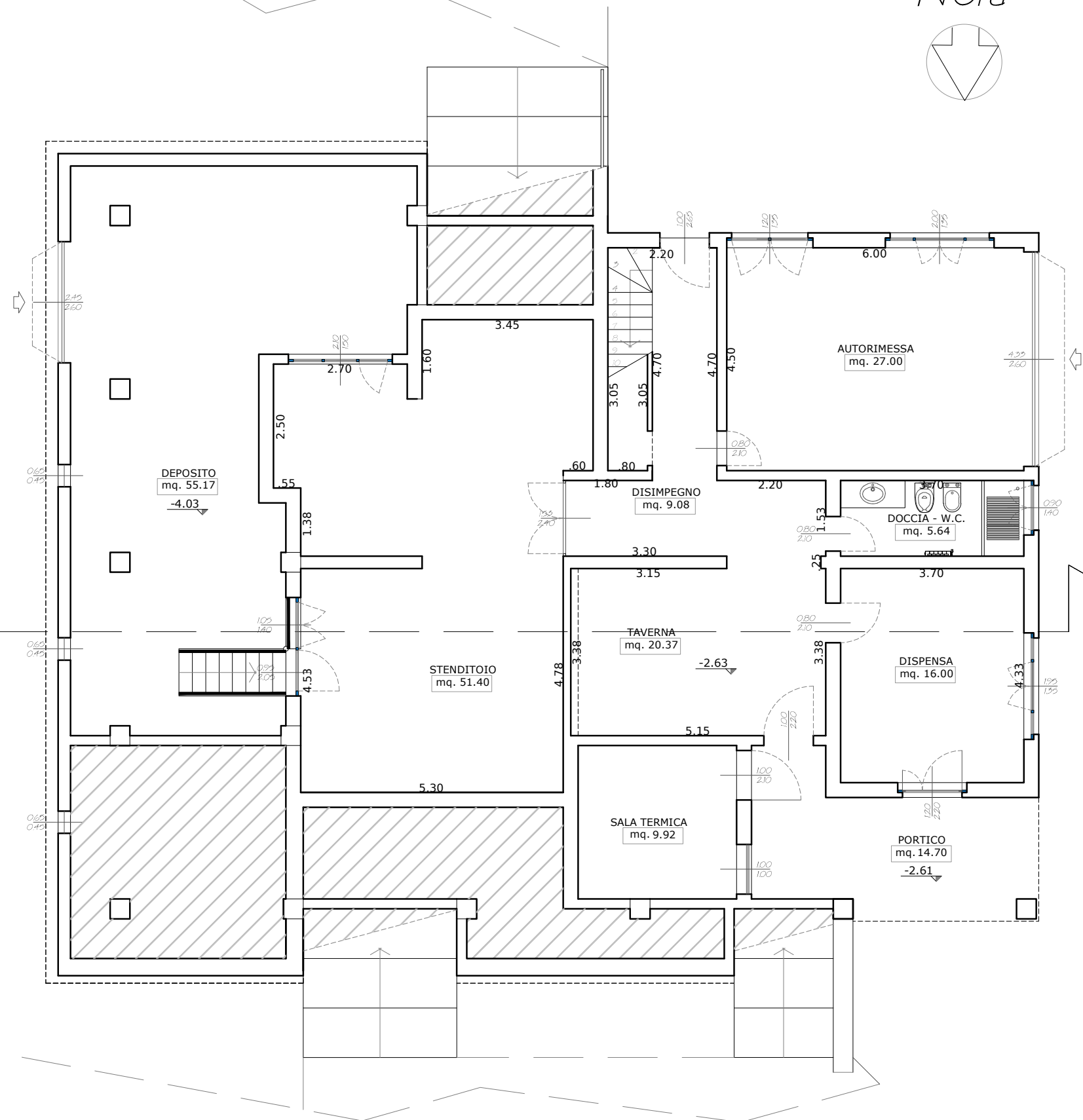
PIANTA DEL PIANO SEMINTERRATO
