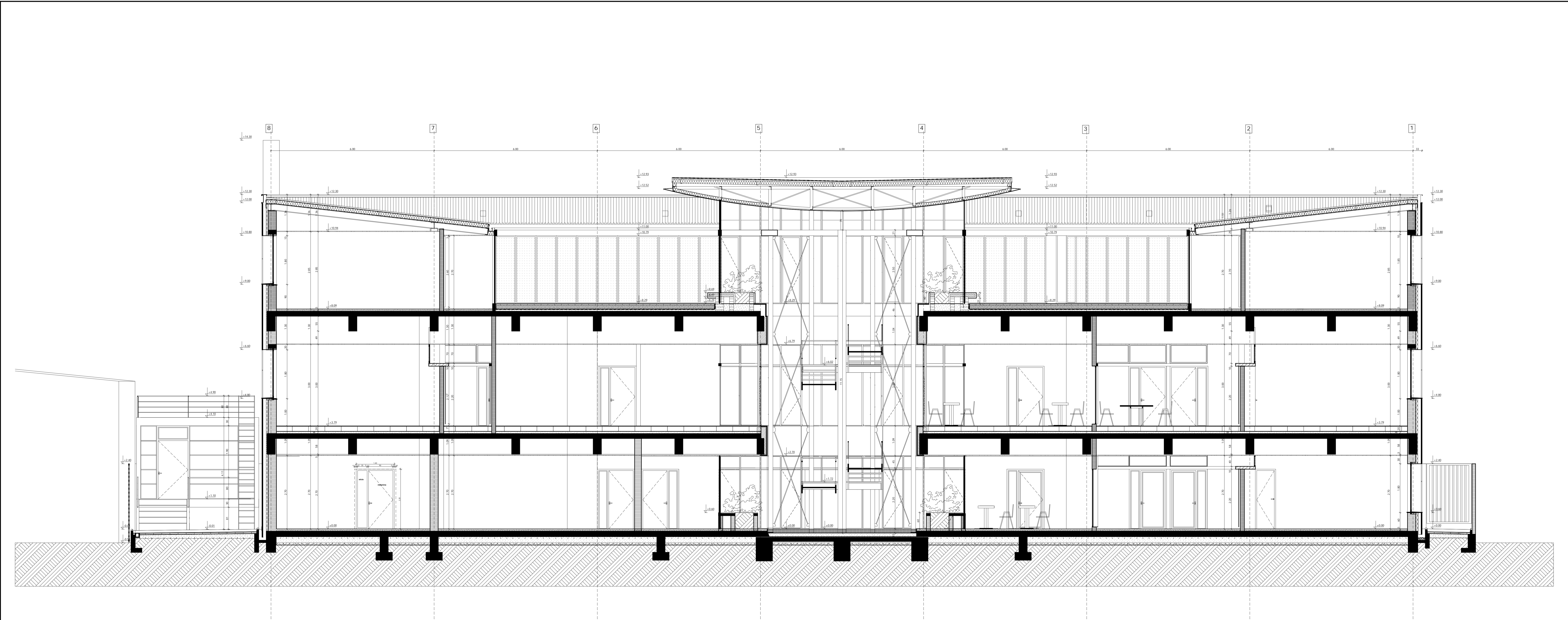
SECTIUNE A-A
