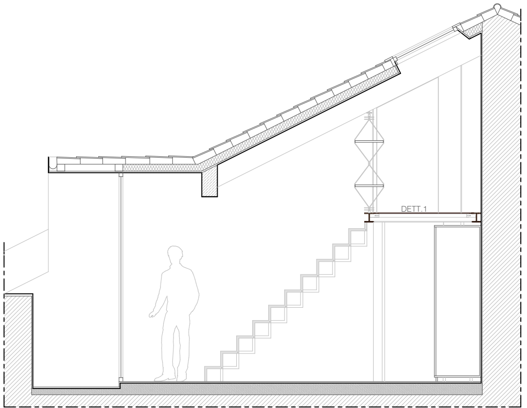
SEZIONE B-B'
