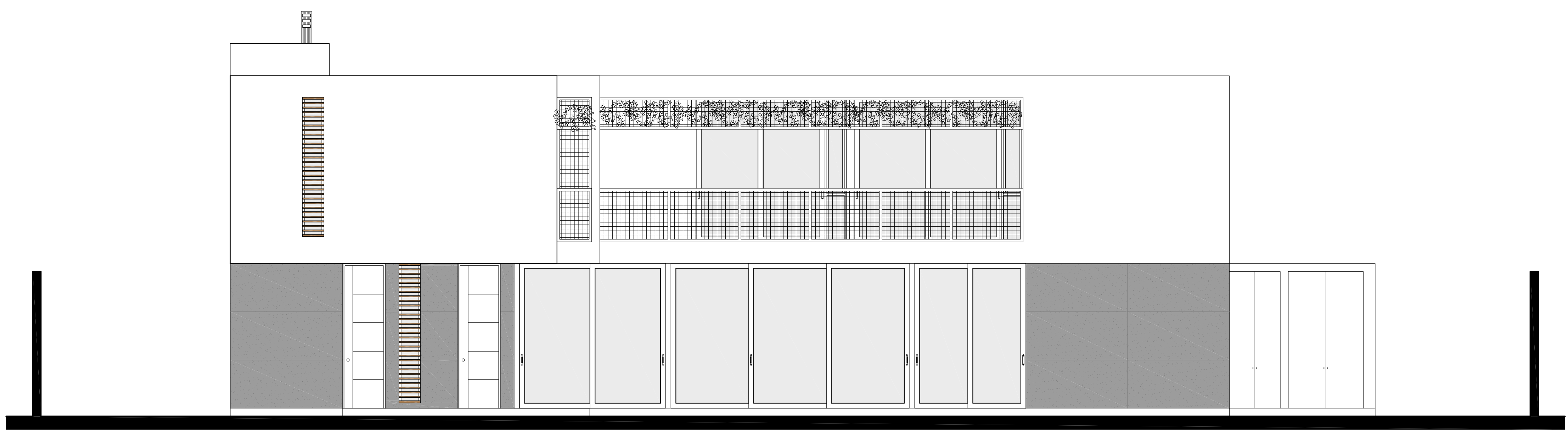
ELEVACIÓN POSTERIOR
