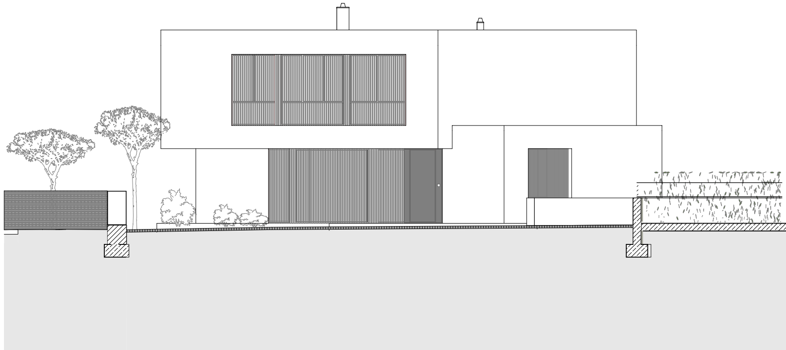
Ansicht Nord-Ost M 1:100
