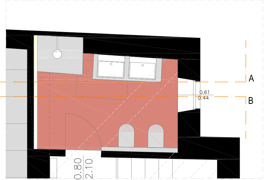
BAGNO SOTTOTETTO SCALA 1:50
