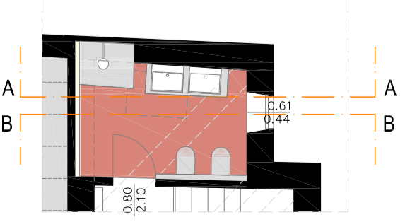
BAGNO SOTTOTETTO SCALA 1:100
