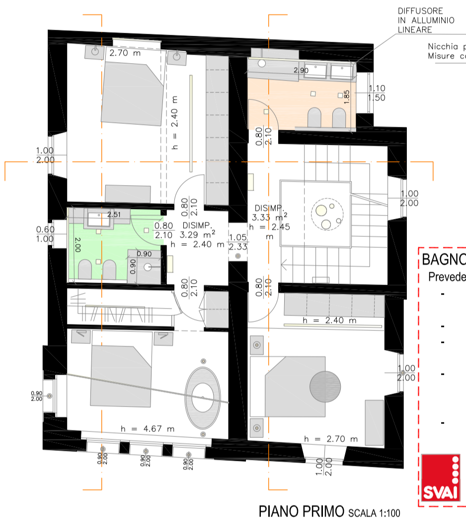
PIANO PRIMO SCALA 1:100
