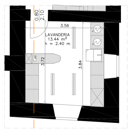
LAVANDERIA SCALA 1:50
