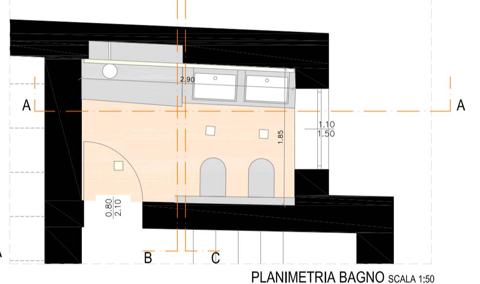
PLANIMETRIA BAGNO SCALA 1:50
