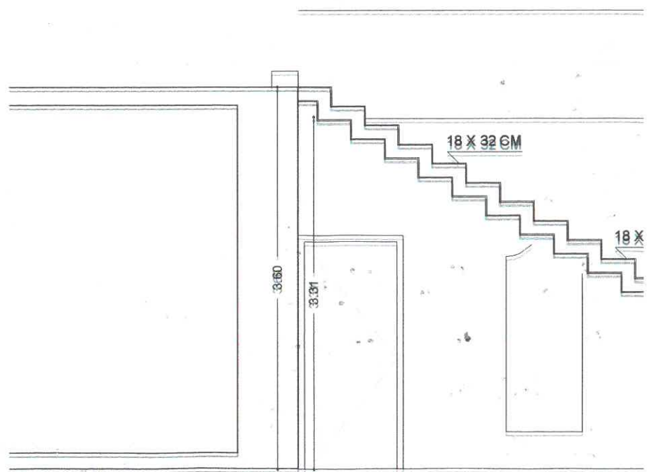
ESCADA EM FERRO escala 1 : 50
