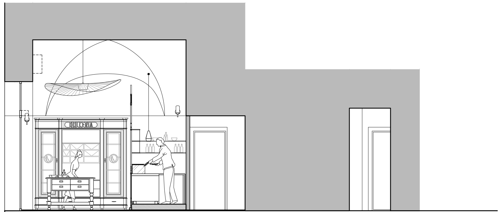
SEZIONE C-C
