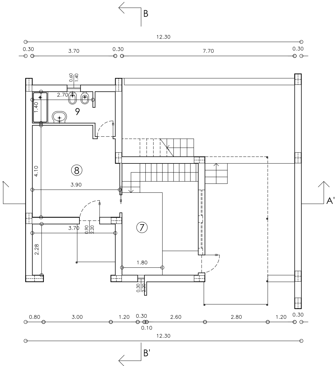
pianta piano primo e coperture (m. 3.25, m. 3.55 e m. 4.25)
