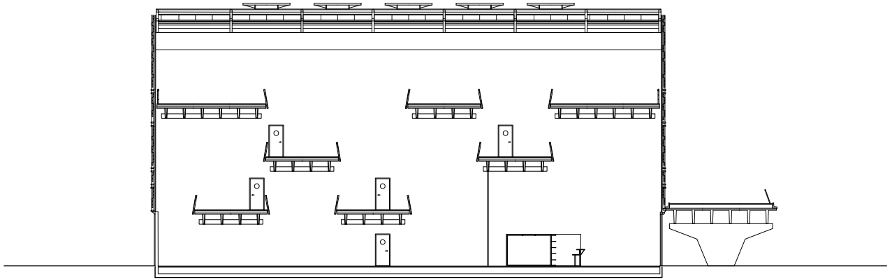
Seccion Longitudinal
