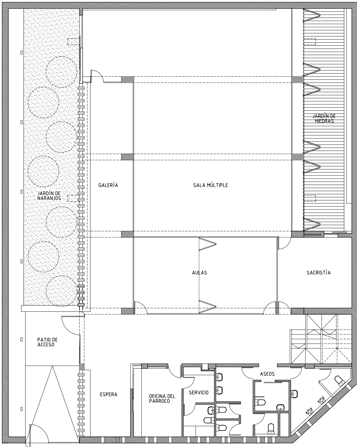
PLANTA DISTRIBUCIÓN
