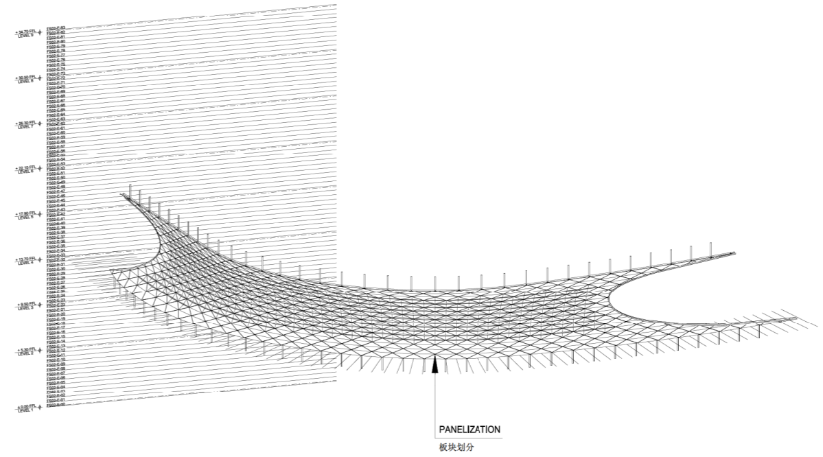
03 幕墙系统02 定位分析图 FS02 Setout SCALE NTS @A0
