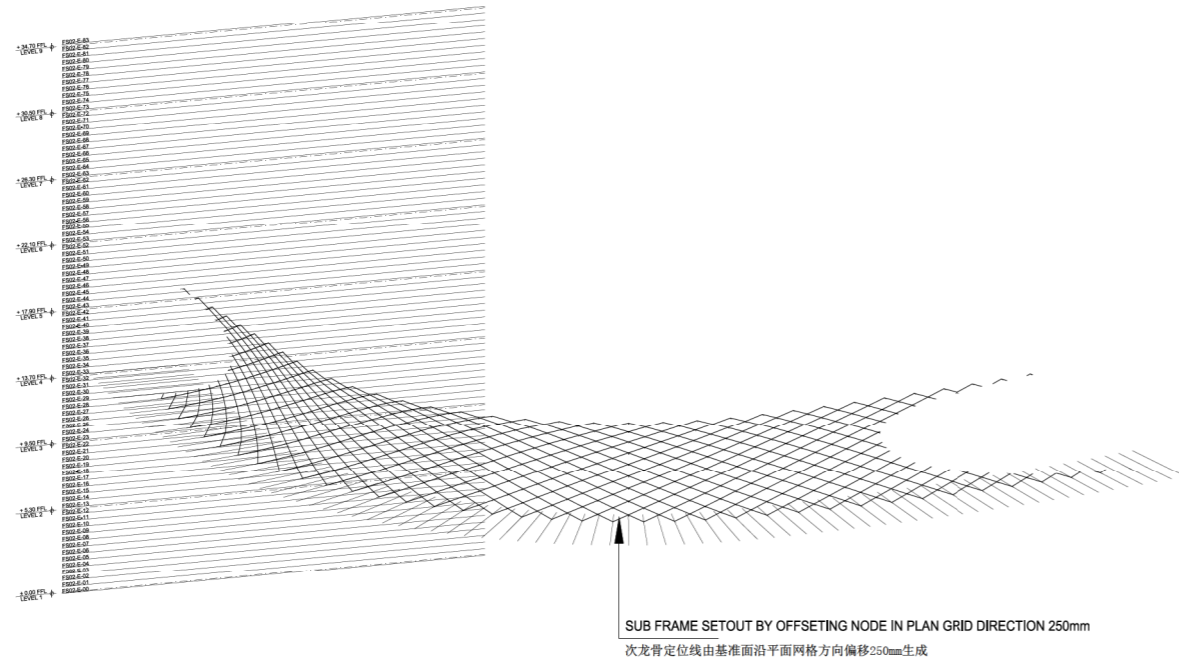
01 幕墙系统02 定位分析图 FS02 Setout SCALE NTS @A0
