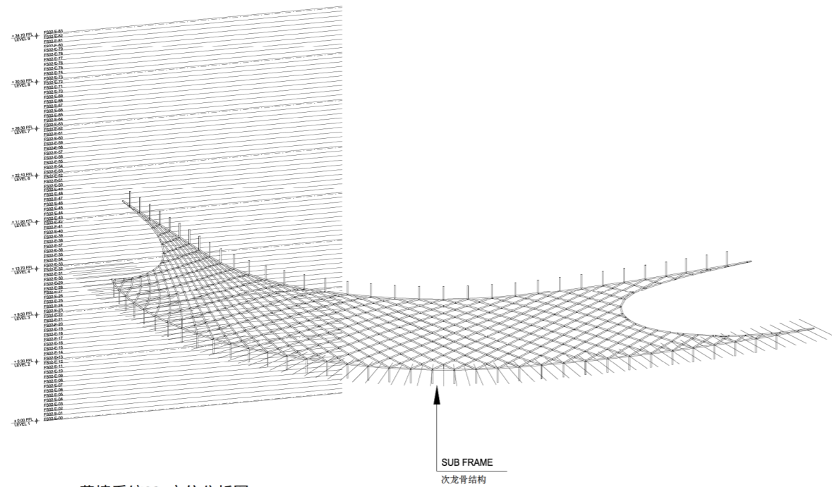
02 幕墙系统02 定位分析图 FS02 Setout SCALE NTS @A0
