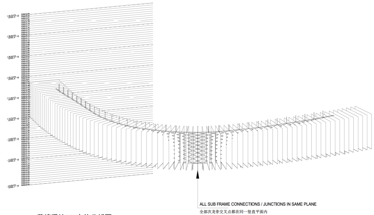
04 幕墙系统02 定位分析图 FS02 Setout SCALE NTS @A0
