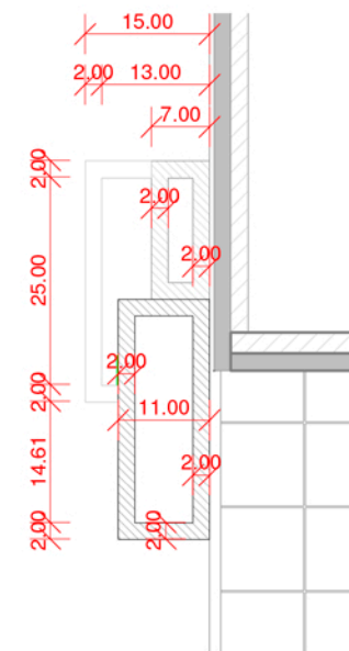
Detalle Sección Y01 1 : 10
