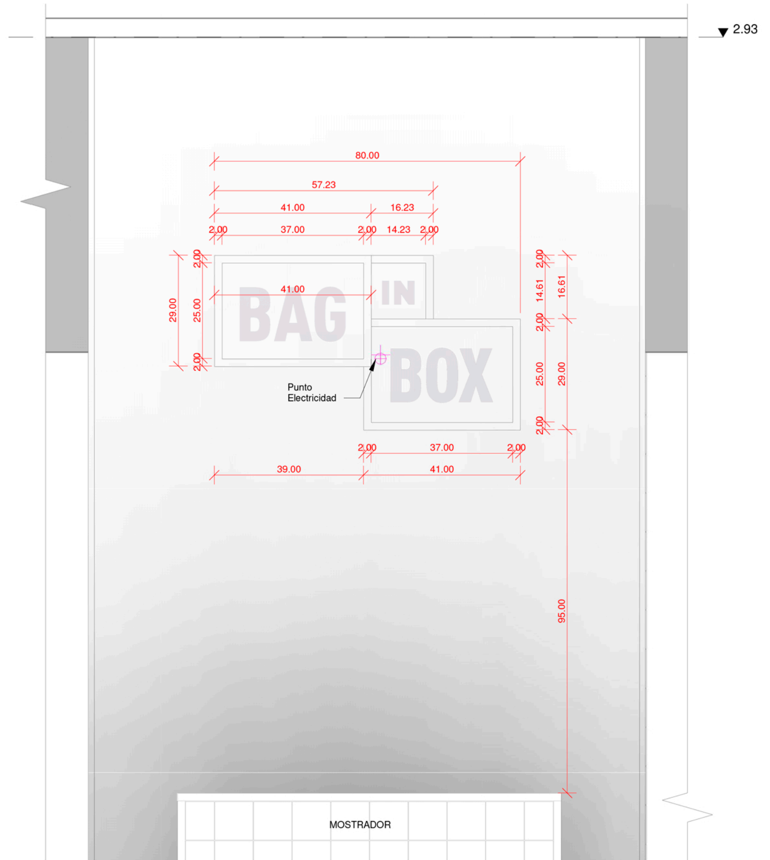
Detalle Frontal 01.1 1 : 10
