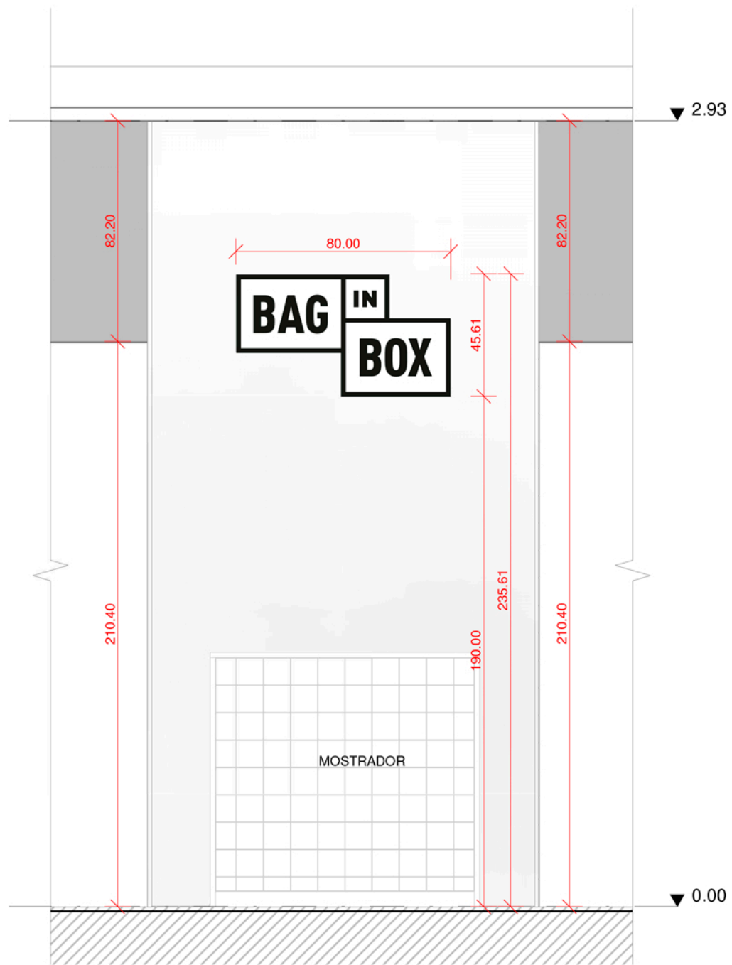
Detalle Frontal 01 1 : 20
