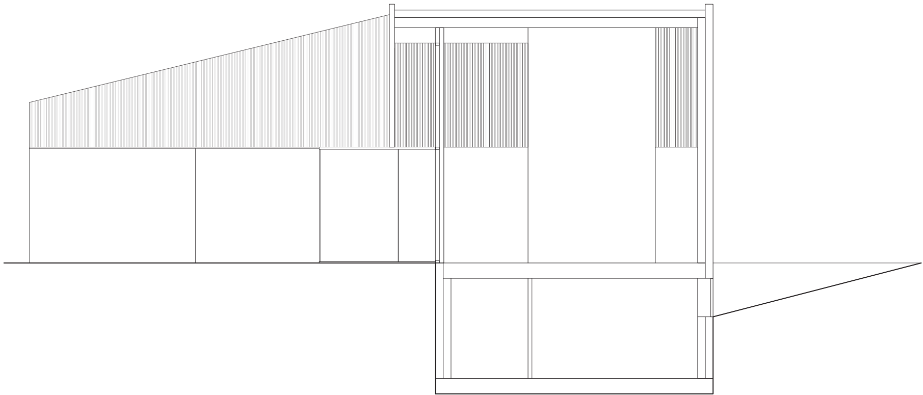
Doorsnede AA
