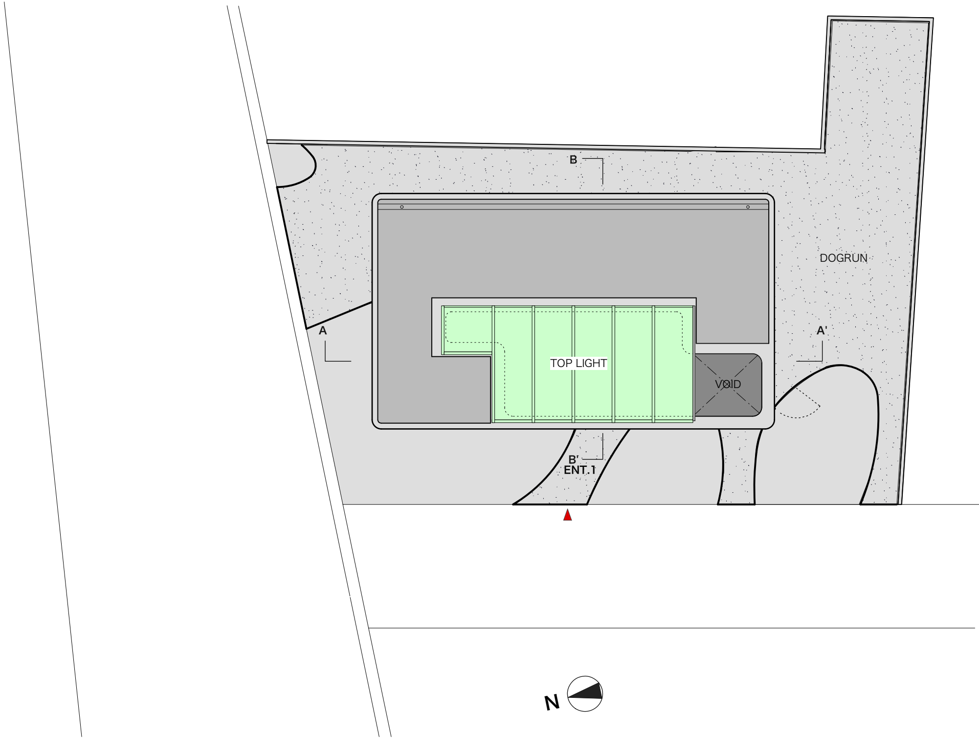
site plan S=1:100
