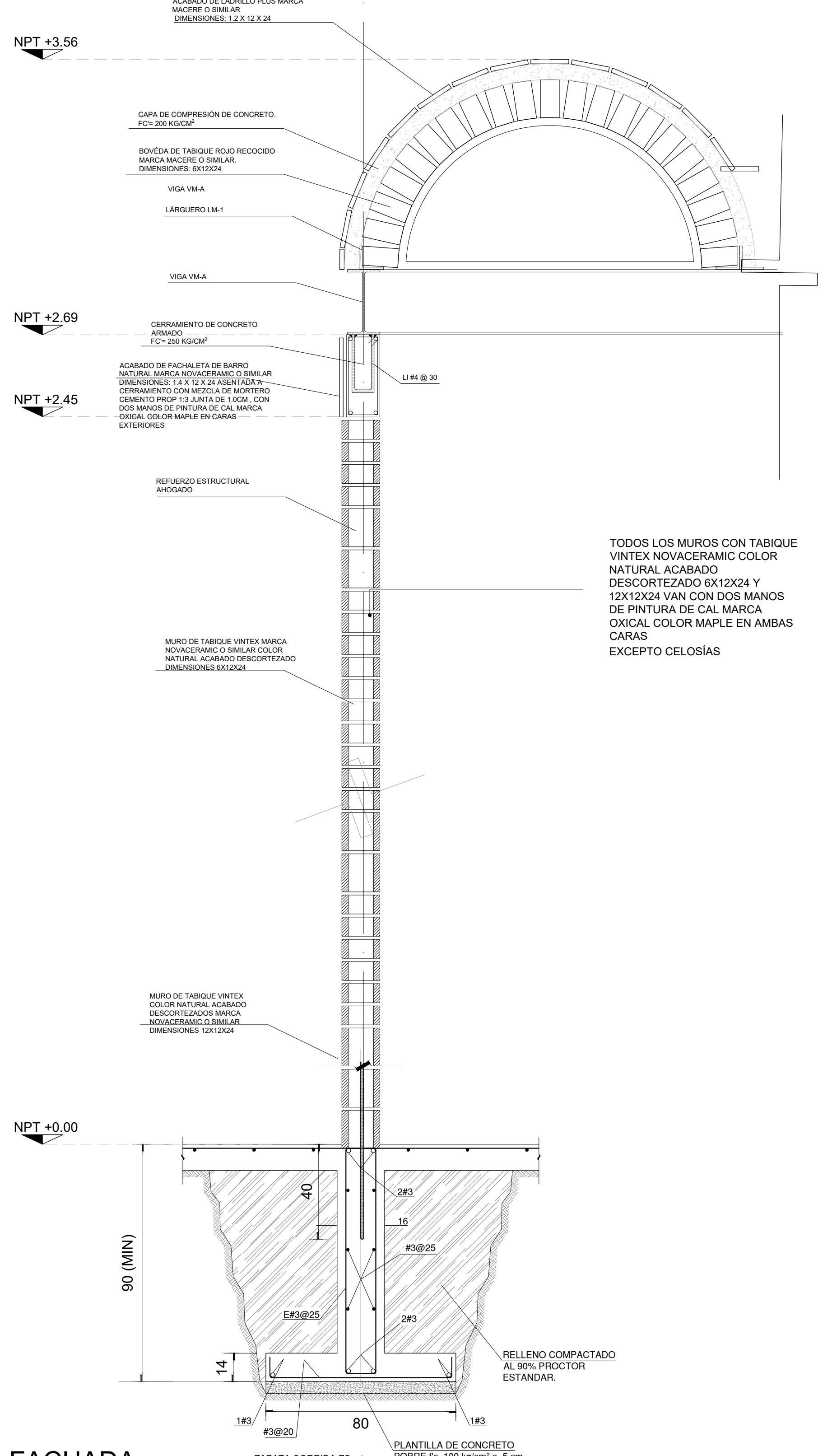
CORTE POR FACHADA CXF C
