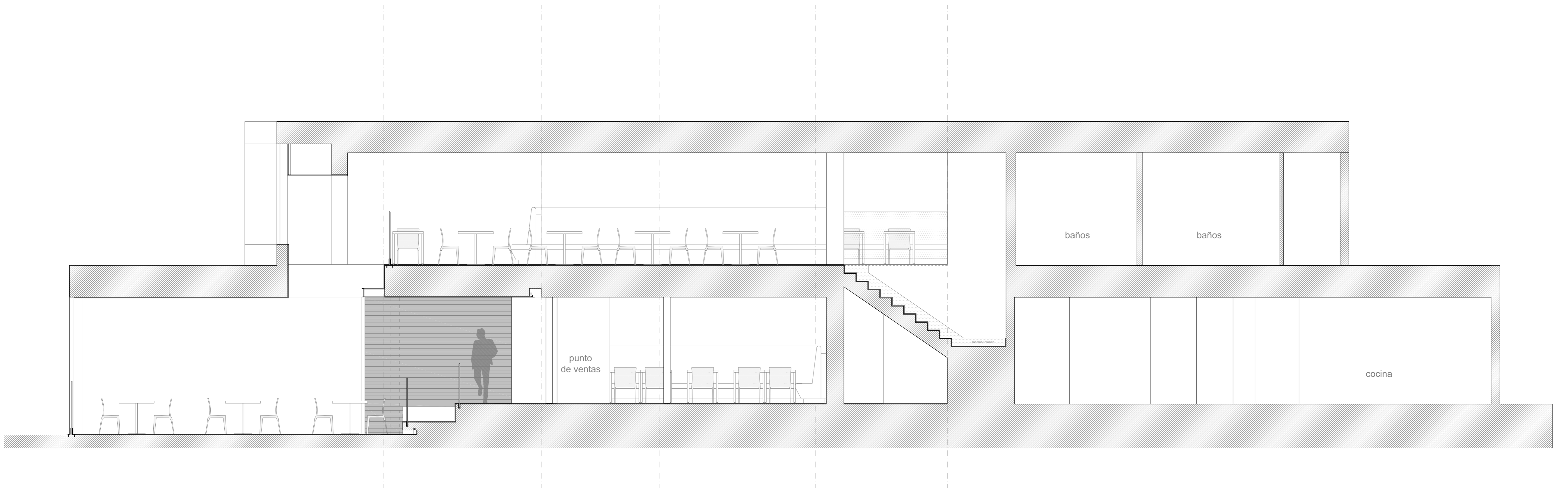
corte X3
