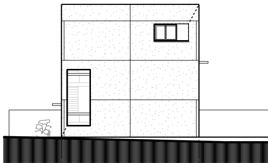
FACADE NORD-OUEST
