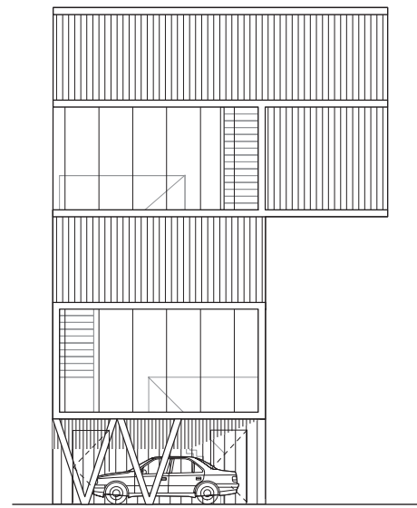
Tuingevel
