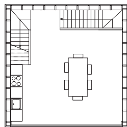
1e verdieping
