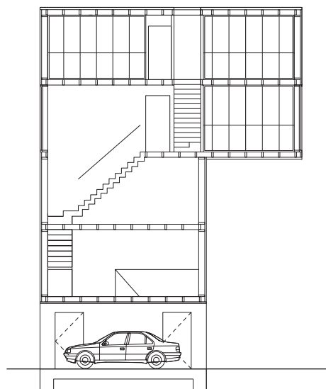
Langsdoorsnede
