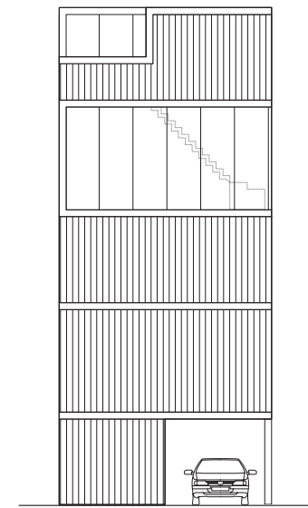
Kopgevel
