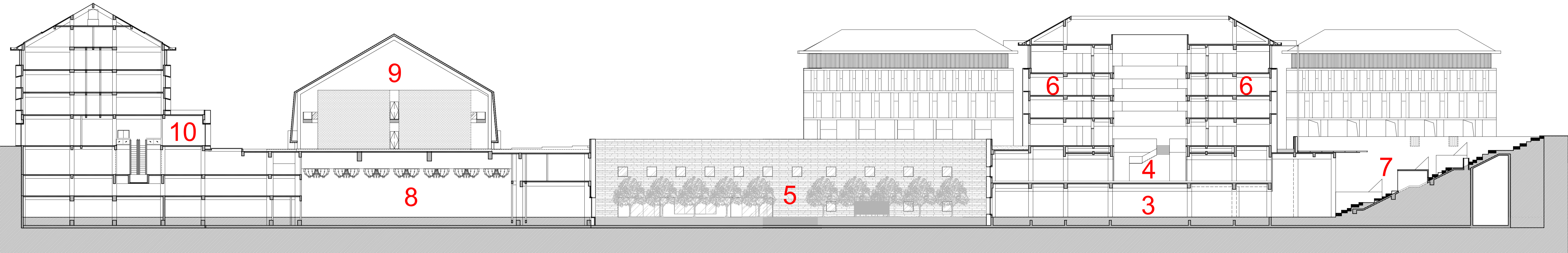
SECTION A-A
