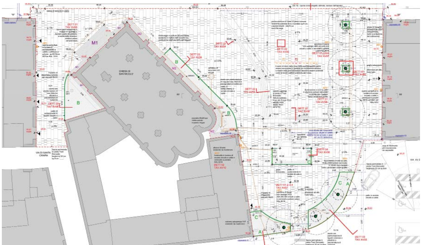
Planimetria progetto esecutivo
