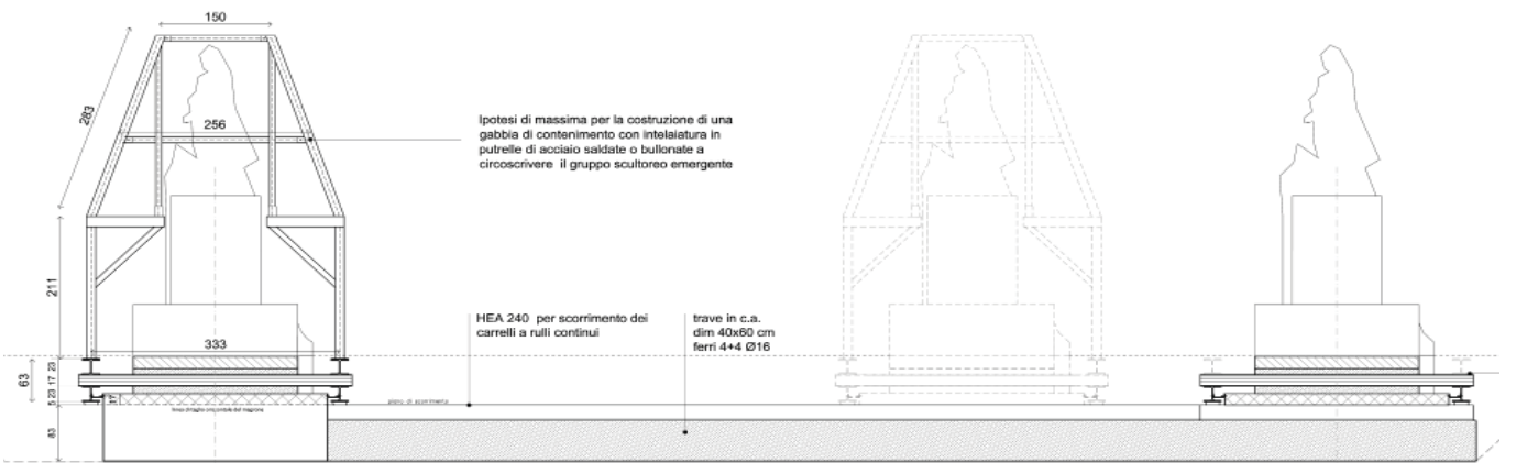
Progetto di spostamento del complesso monumentale
