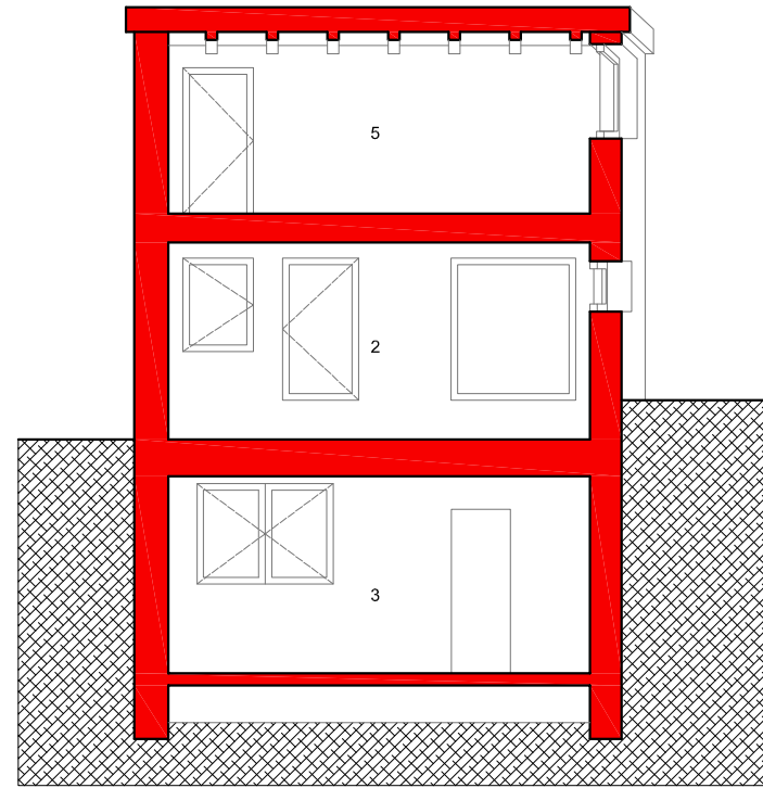
SEZIONE D-D
