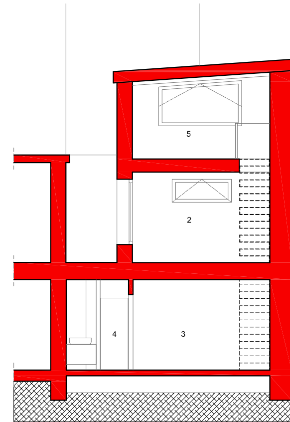
SEZIONE E-E
