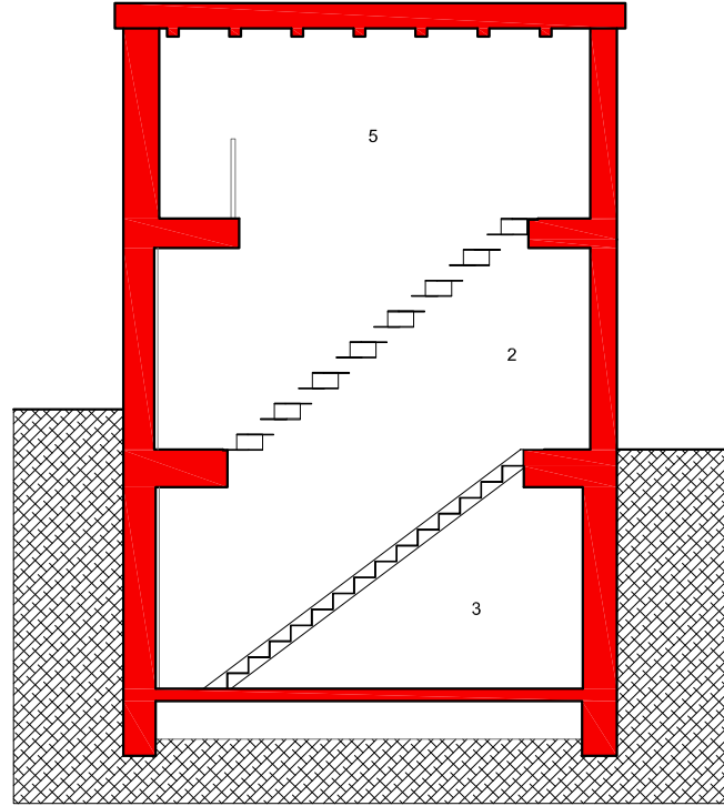
SEZIONE B-B
