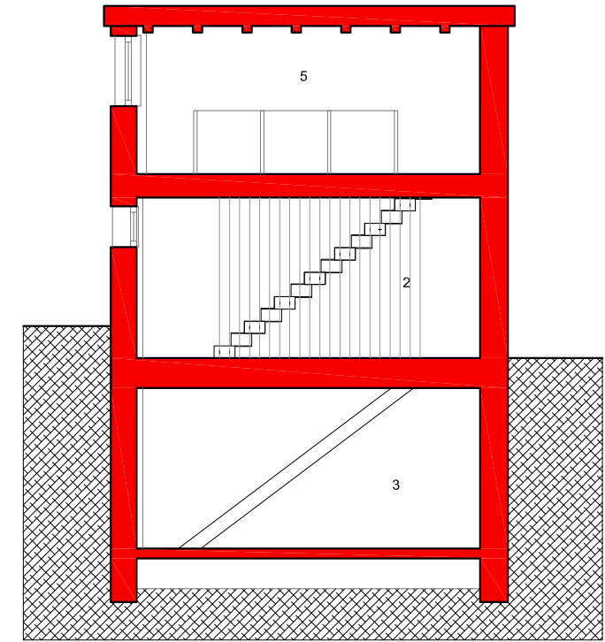
SEZIONE A-A
