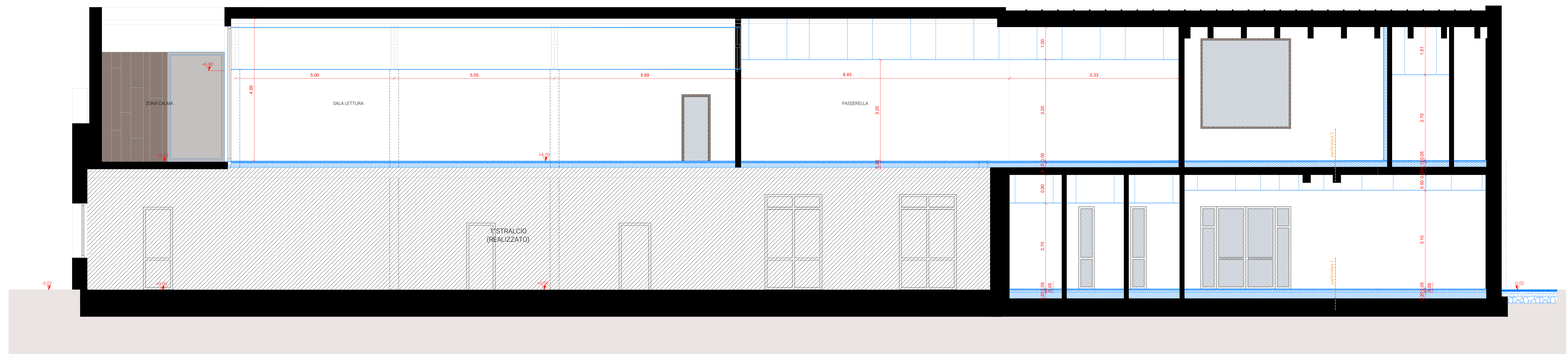
sezione E-E scala 1:50
