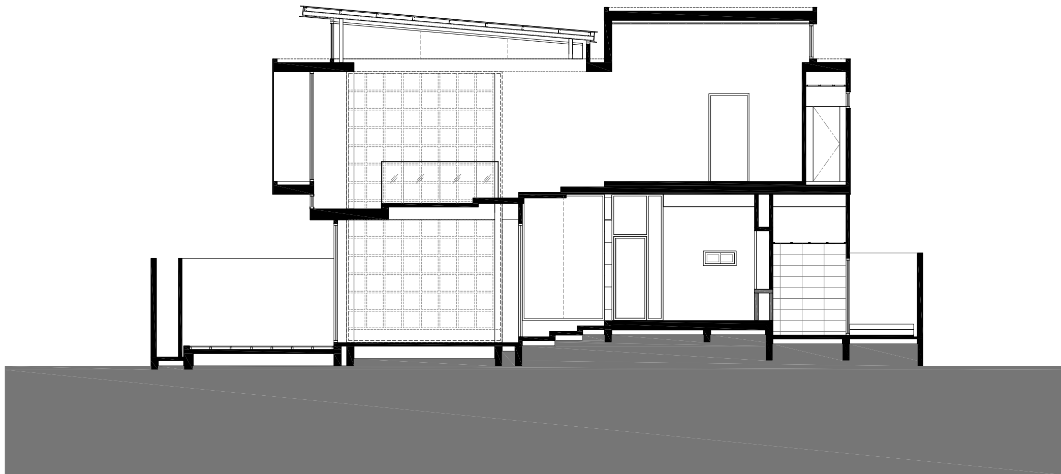
A-A SECTION
