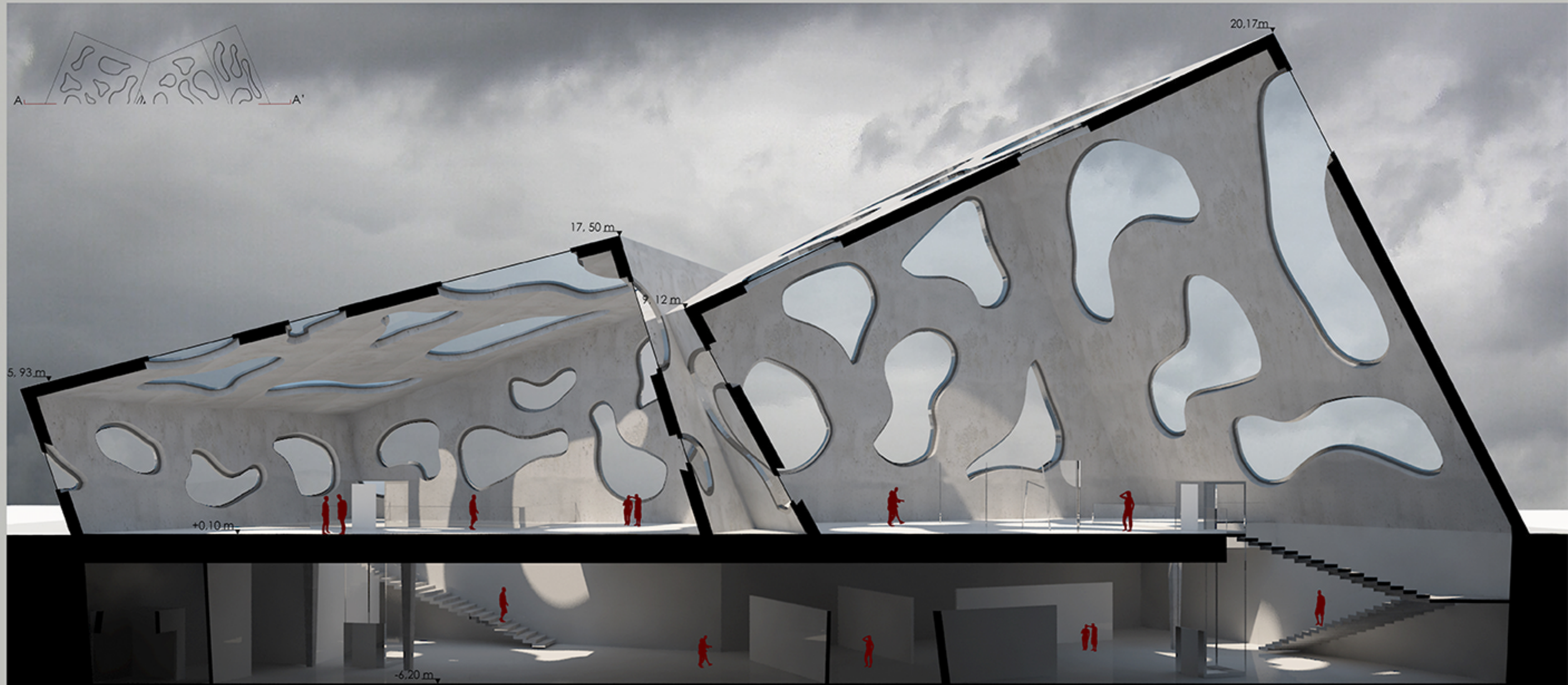
Sezione A - A' // Section A - A'
