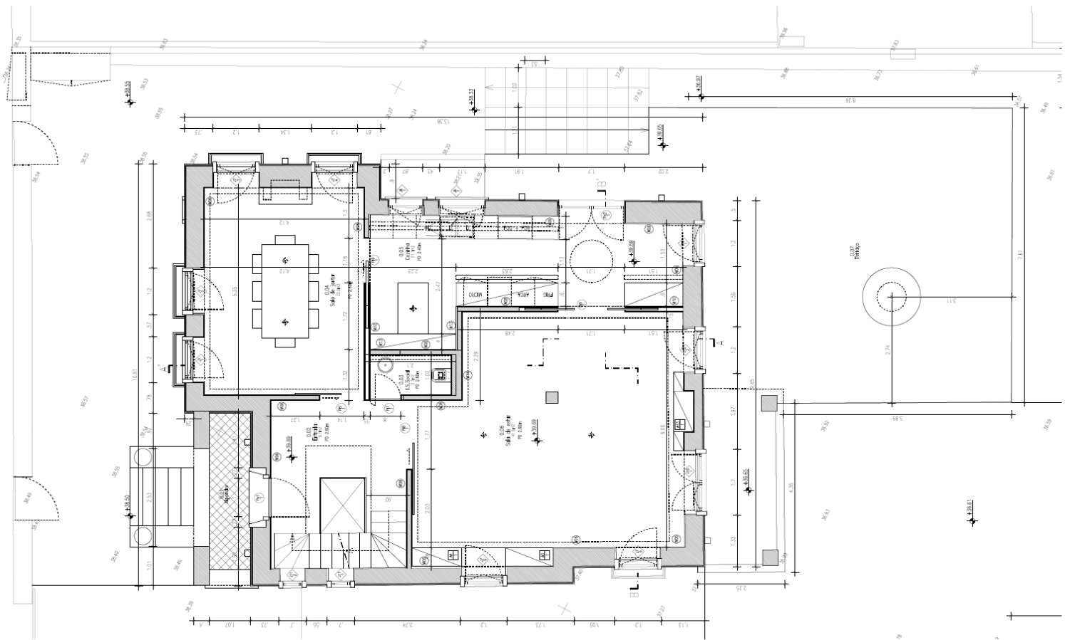
PLAN. 00 (RD - 0) ES. 1/50
