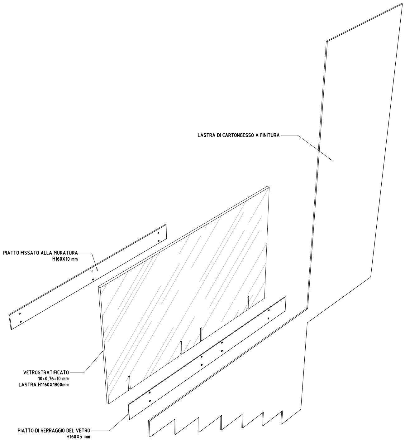
DETTAGLIO PROSETTICO DEGLI ELEMENTI PRINCIPALI COMPONENTI IL PARAPETTO IN VETRO
