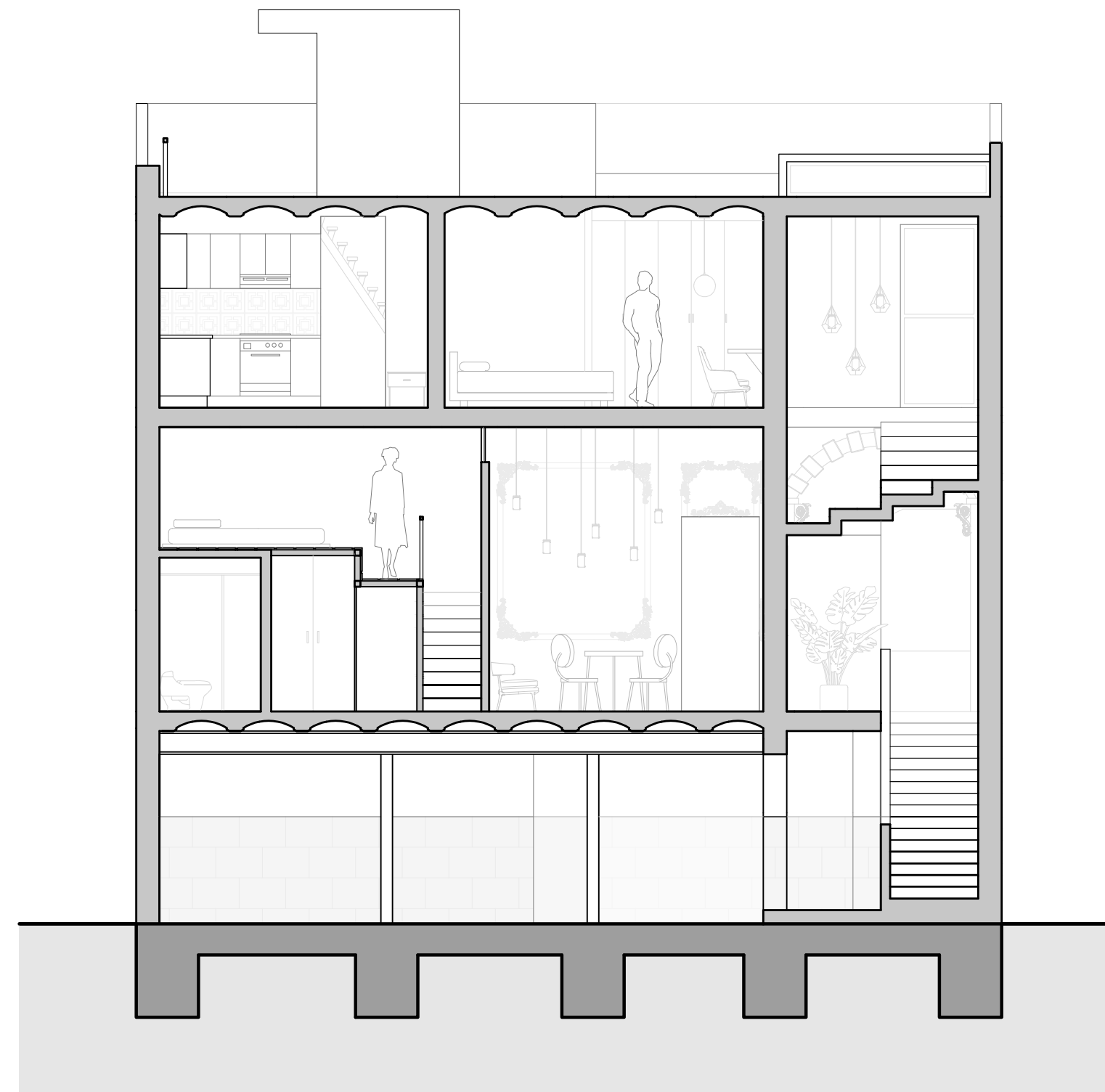
MM34 | MAR MEDITERRANEO 34 SECCIÓN TRASVERSAL | CROSS SECTION
