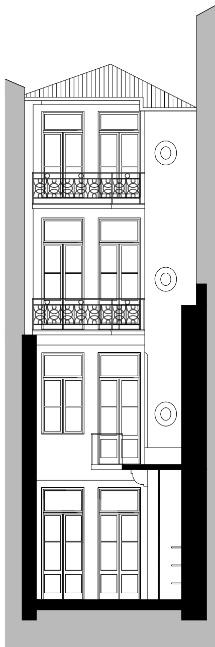
ALÇADO POSTERIOR (A2)
